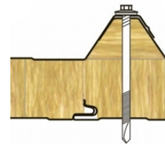
Крепление типа Кровельный замок
