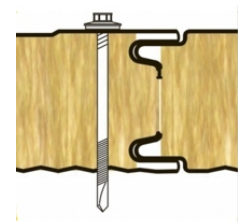
Крепление типа Z-LOCK
