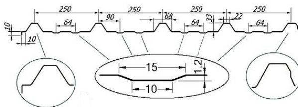
Профиль кровельной панели
